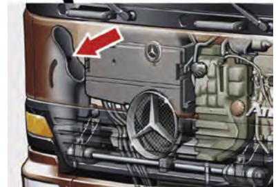
Imagen 114. Lugar de proyección de CO 2 en el compartimento camión de camiones (Flecha)
