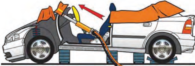
Imagen 284. Abatimiento de salpicaderos
