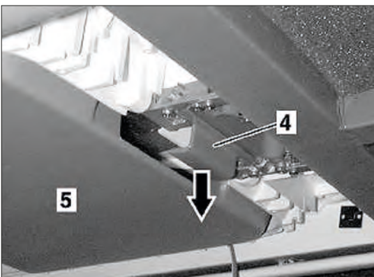
Imagen 357. Ejemplo apertura de trampillas en autobús urbano (3)
