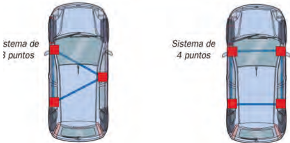
Imagen 142. Estabilización de un vehículo sobre sus ruedas
