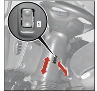
Imagen 334. Regulación de la altura e inclinación del volante
