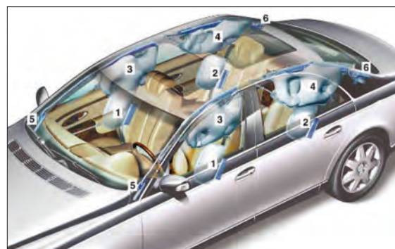
Ejemplo Disposición de los airbags en un Mercedes
