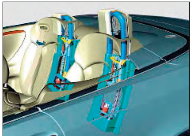
Imagen 315. Arco protector extensible
