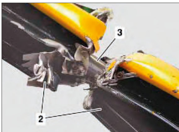
Imagen 246. Montante A (2) y tubo de refuerzo (3)
